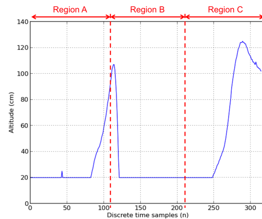
(d) Altitude data samples from sonar
